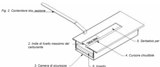
Fig. 2. Contenitore bio- sezione
