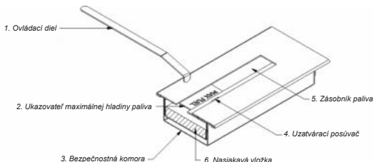
Obr. 2: Nádoba na biopálivo – prierez
