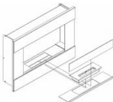
Obr. 3: Způsob montáže skla na biokrbch Alpha, Bravo, Bravo 2, Charlie, Charlie 2, Delta, Delta 2, Golf, Quat
