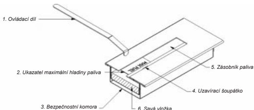
Obr. 2: Nádoba na biopalivo – průřez
