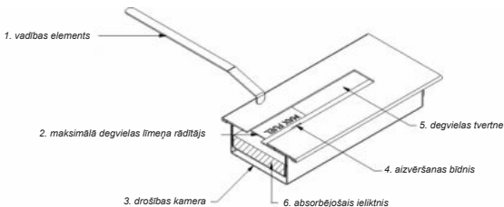
2. attēls. Biokonteiners – šķērs griezumā
