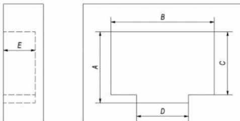
10.sz.kép: A bio kandalló külse méretei
