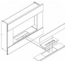
3 pav. Biožidinių „Alpha“, „Bravo“, „Bravo 2“, „Charlie“, „Charlie 2“, „Delta“, „Delta 2“, „Golf“ ir „Quat“ stiklo montavimo būdas
